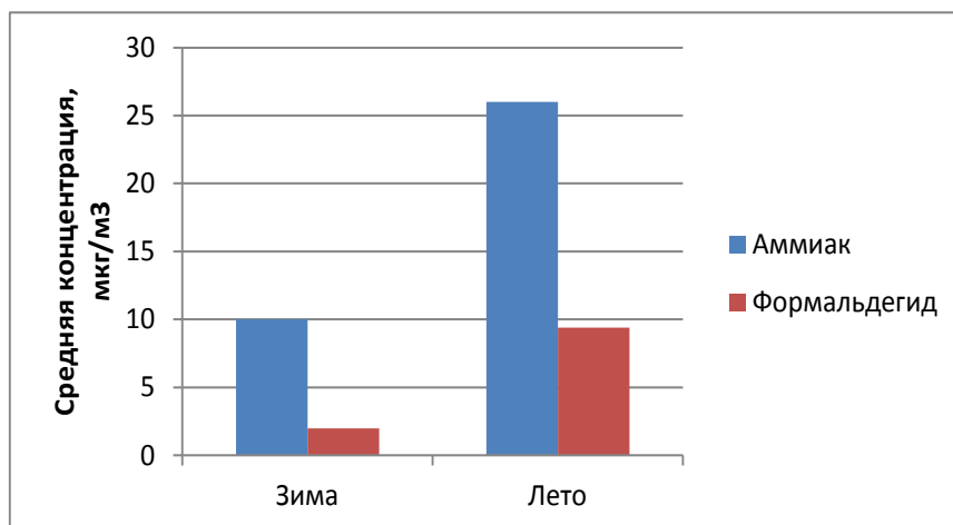
Рисунок 4.20 – Сезонные изменения концентраций специфических загрязняющих веществ
