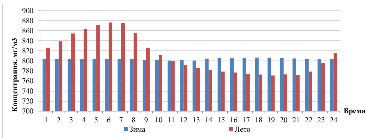
Рисунок 4.27 – Суточный ход концентраций диоксида углерода в атмосферном воздухе Березинского заповедника
