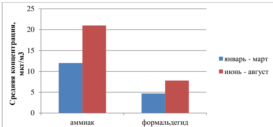
Рисунок 4.3 – Сезонные изменения концентраций специфических загрязняющих веществ
