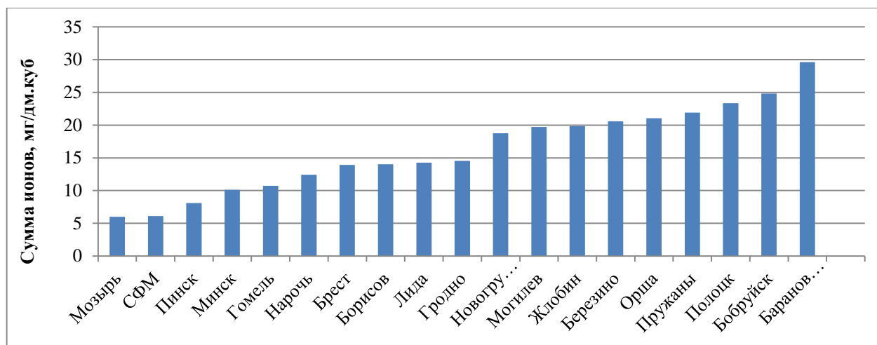
Рисунок 4.28 – Минерализация атмосферных осадков в городах Беларуси в 2013 г.
