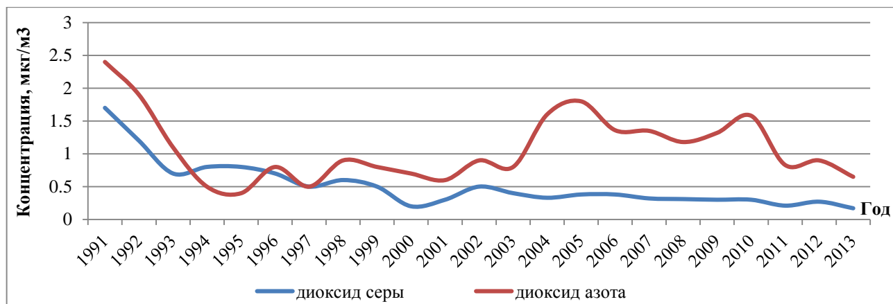
Рисунок 4.26 – Изменение среднегодовых концентраций диоксида серы и диоксида азота ( \text{мкг/м}^3 ) в воздухе Березинского заповедника
