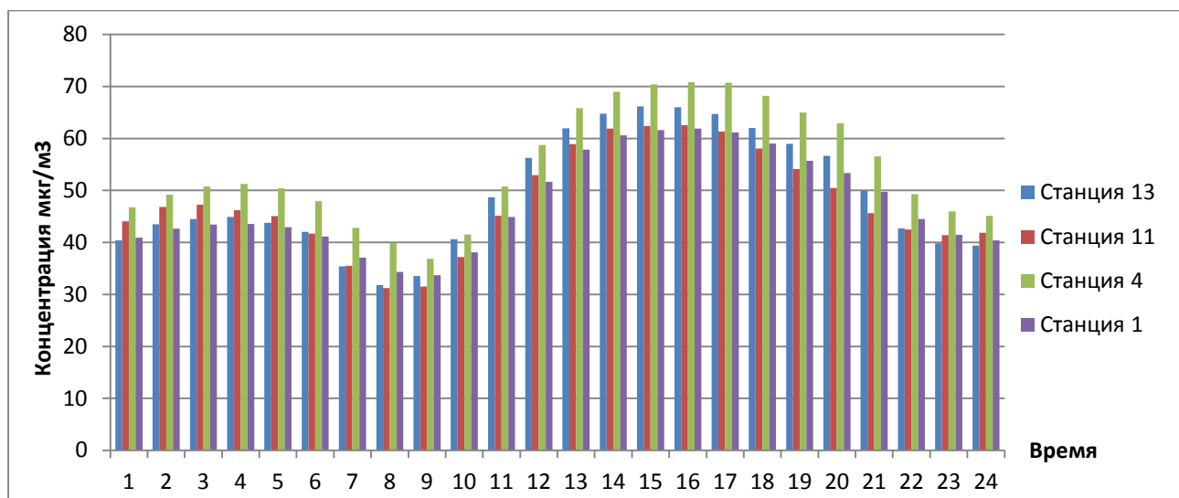
Рисунок 4.5 – Суточный ход концентраций приземного озона в 2013 г.
