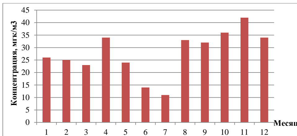
Рисунок 4.14 – Внутригодовое распределение среднесуточных концентраций ТЧ-10 в атмосферном воздухе г. Гомель (станция №14)
