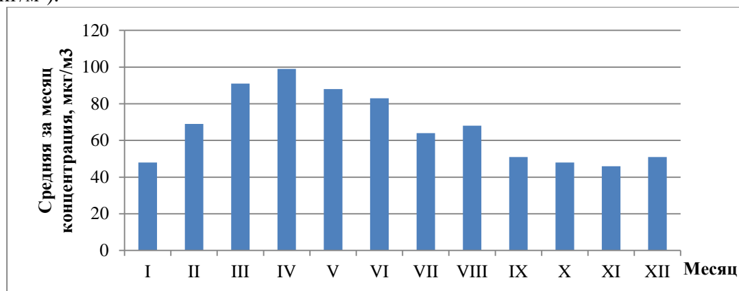
Рисунок 4.23 – Внутригодовое распределение среднемесячных концентраций приземного озона
