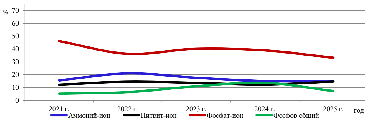
Рисунок 2.48 – Динамика вклада биогенных веществ в загрязнение воды притоков р. Днепр за период 2021 – 2025 гг.
