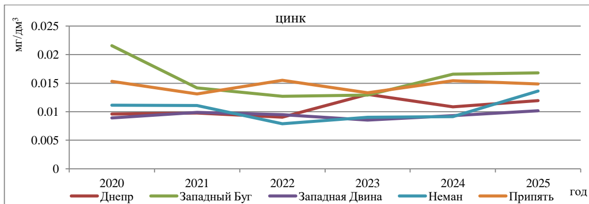
Рисунок 2.83 – Среднегодовые концентрации цинка за период 2020 – 2025 гг.
